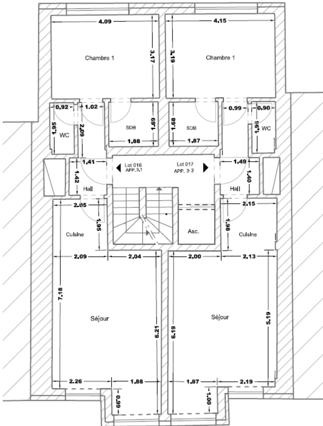
ETAGE 3
