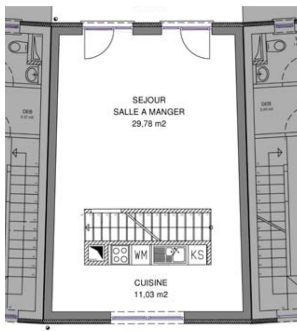
1 er étage
