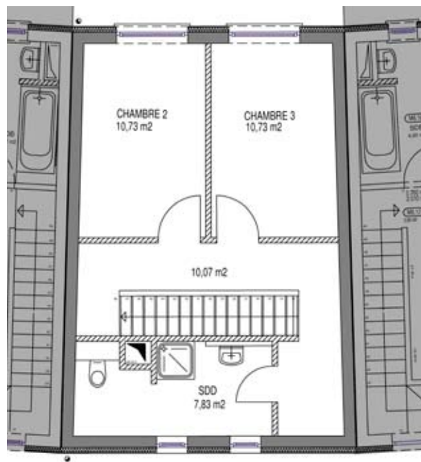
3 e étage
