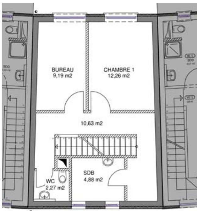
2 e étage
