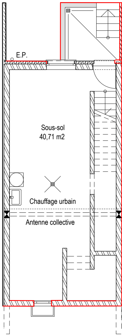
SOUS-SOL
