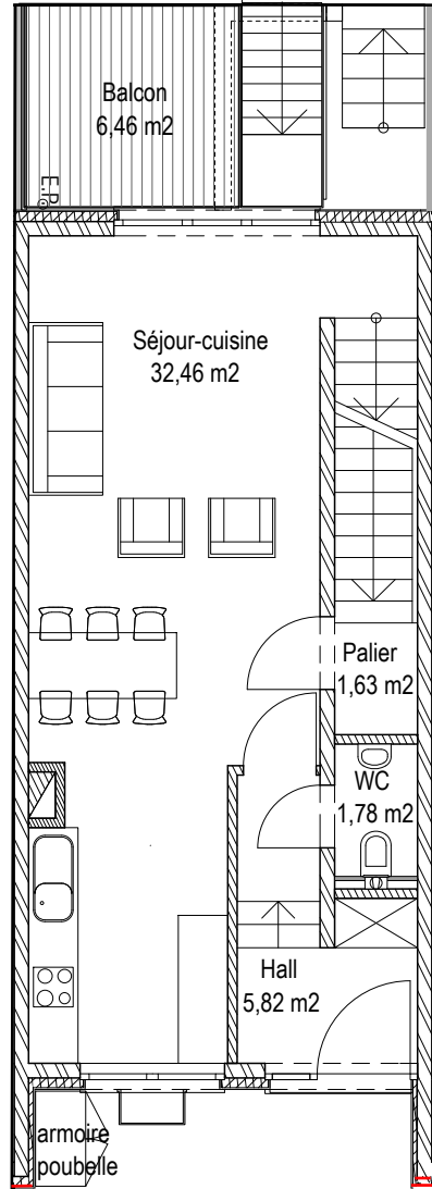
REZ-DE-CHAUSSEE
