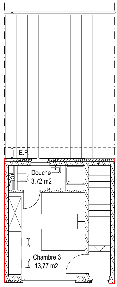
ETAGE 2
